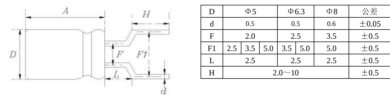
引线切脚成型 G 图
