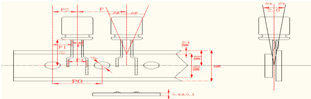
编带外型尺寸 B 图
